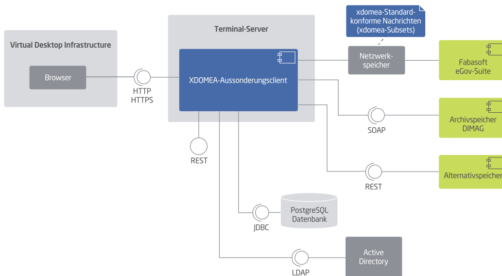
Abbildung 1: Technischer Kontext und Schnittstellen
